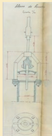
Vista en alzado de la fuente. Fondo documental AMS
